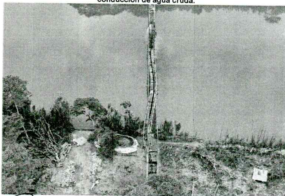
Foto N°11: Tramo de estructura metálica de soporte de tubería en el cruce del río para la conducción de agua cruda.
